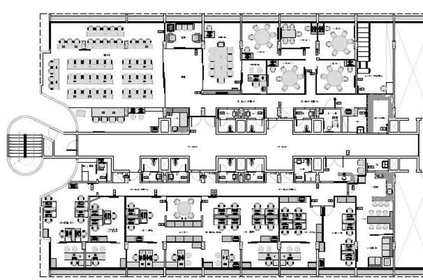
PLANTA DE SINALIZAÇÃO CONSELHO FEDERAL DE NUTRICIONISTAS 1/75
